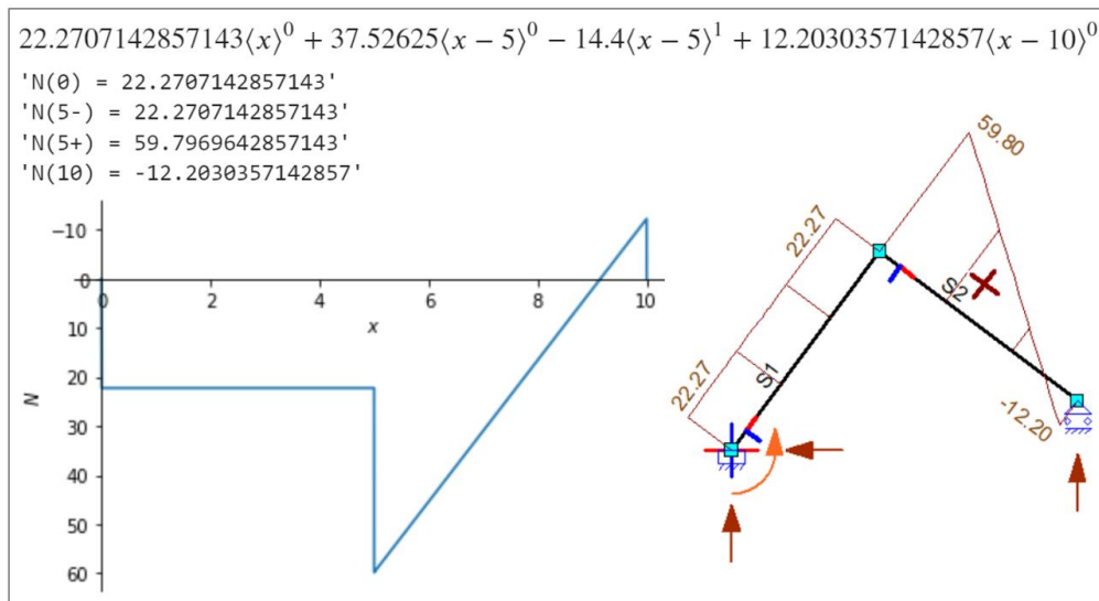
figuur 57: De normaalkrachtenlijn volgens de Macaulay methode links en Matrixframe rechts(zelfgemaakt).
