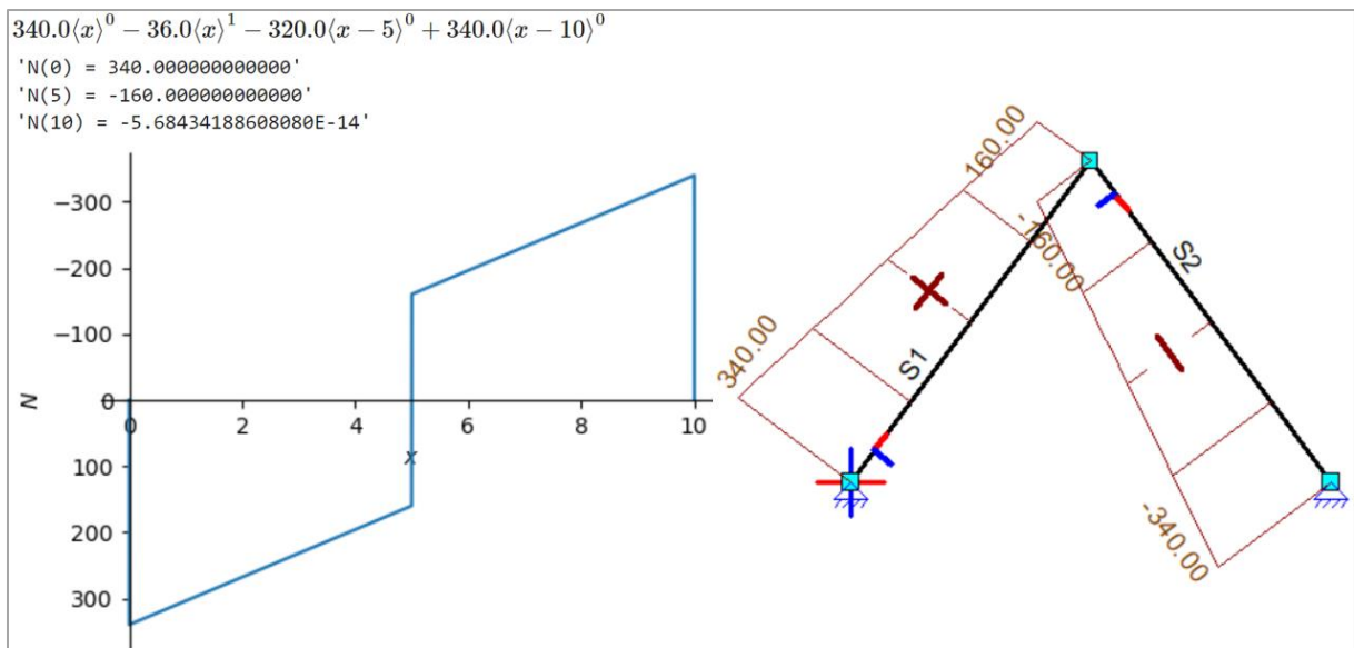
figuur 50: Normaalkrachtenlijn volgens het model links en Matrixframe rechts.
