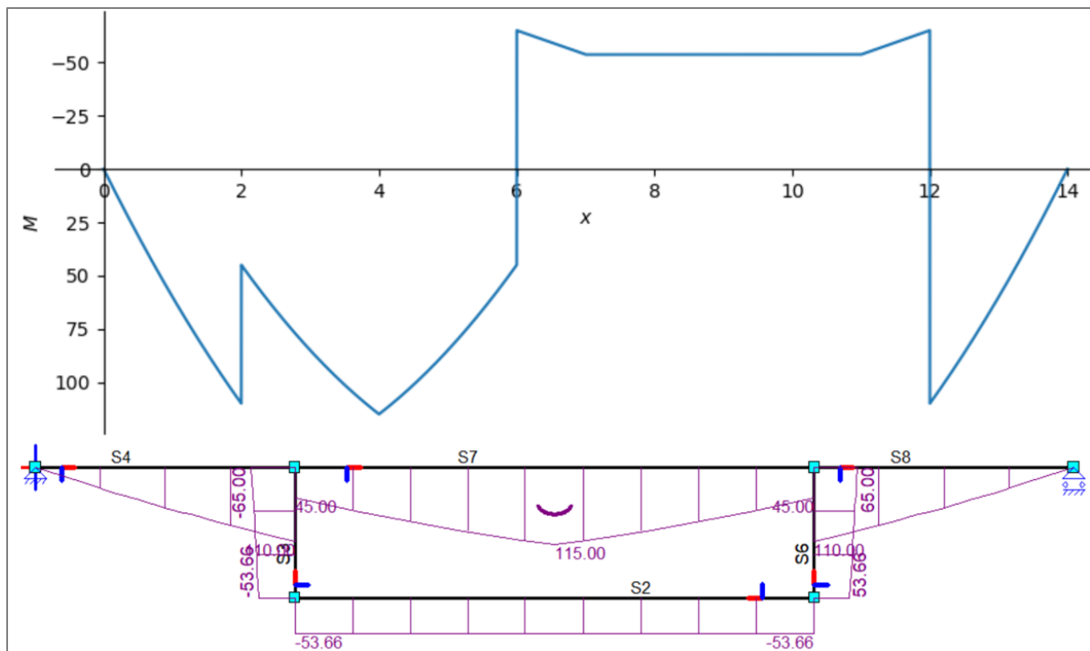
figuur 82: Momentenlijn volgens het model boven en Matrixframe onder.
