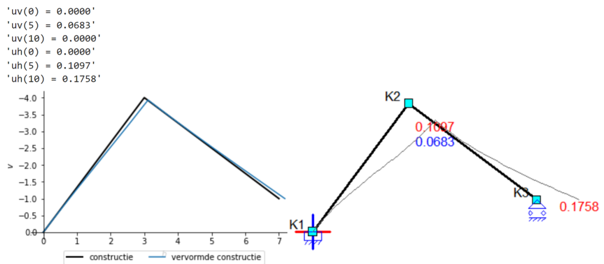
figuur 60: De knooppunt verplaatsingen volgens Matrixframe. Blauw is verticaal en rood is horizontaal.
