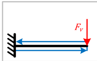
figuur 94: Retour over ingeklemde ligger met een puntlast op het uiteinde.
