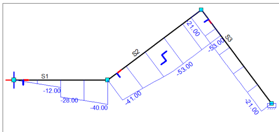
figuur 43: Dwarskrachtenlijn volgens Matrixframe.
