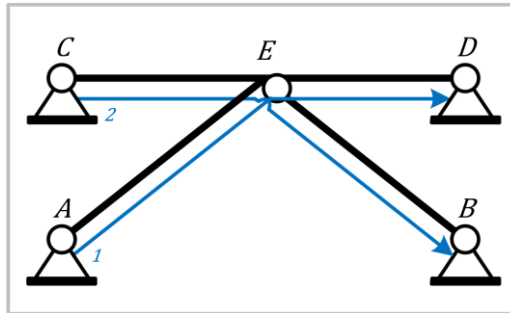
figuur 33: Scharnierverbinding net na aansluitpunt.
