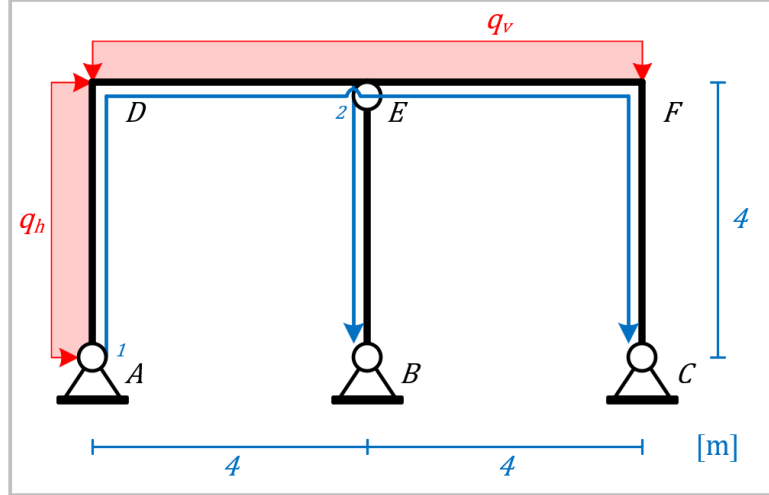
figuur 69: Statisch onbepaalde langshal.
