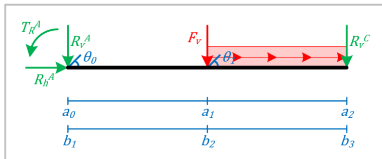
figuur 55: Overzichtsschema behorende bij figuur 54..
