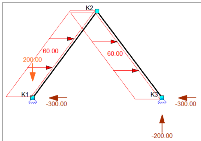
figuur 49: Resultaten voor de reactiekrachten volgens Matrixframe.
