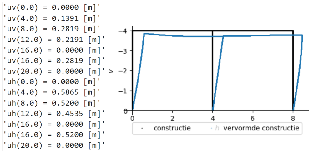
figuur 75: Vervormingen volgens het model.
