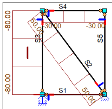
figuur 88: Normaalkrachtenlijn volgens Matrixframe.
