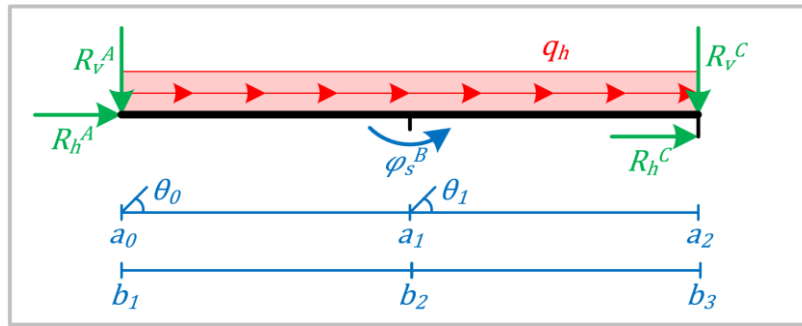
figuur 48: Overzichtsschema behorende bij figuur 47.
