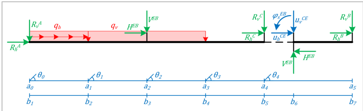
figuur 70: Overzichtsschema behorende bij figuur 69.
