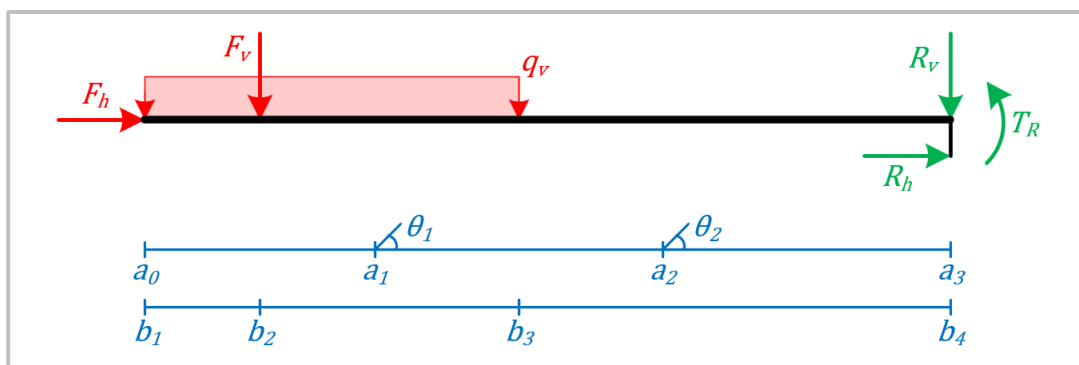
figuur 38: Overzichtsschema behorende bij figuur 37.
