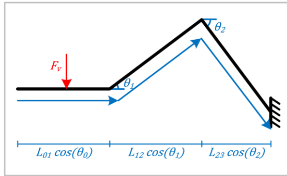
figuur 90: ingeklemde ligger met een knik in punt 1 en 2 dat belast wordt door F_v .
