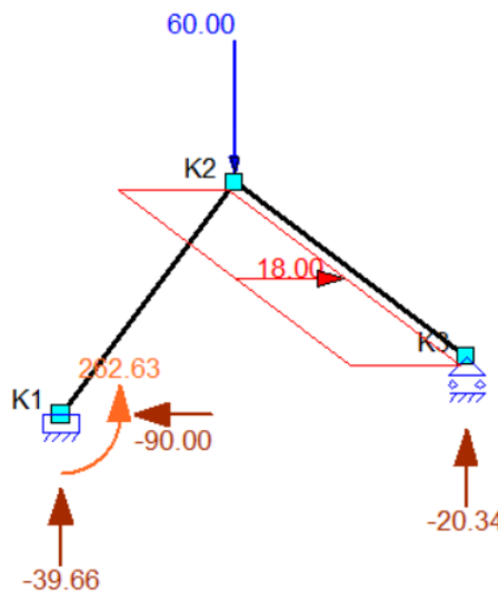
figuur 56: Reactiekrachten in Matrixframe.
