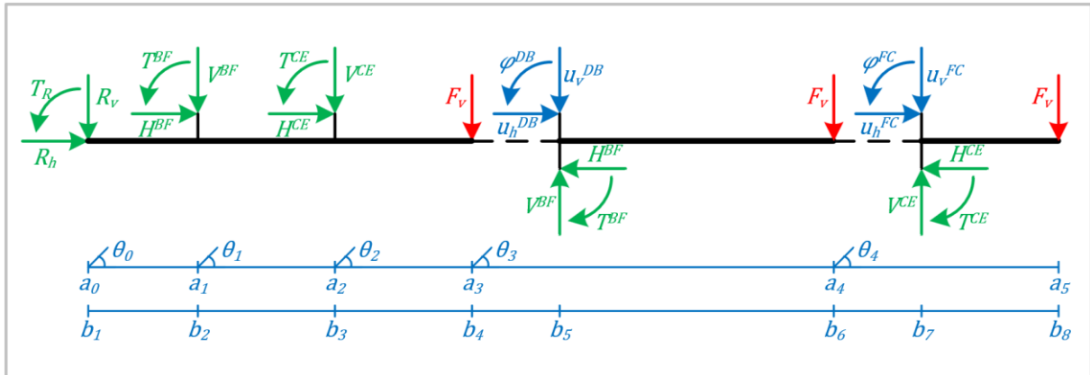
figuur 62: Overzichtsschema behorende bij figuur 61.
