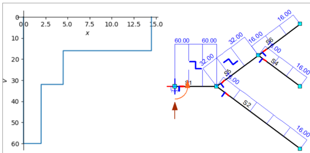
figuur 65: Dwarskrachtenlijn volgens het model links en Matrixframe rechts.
