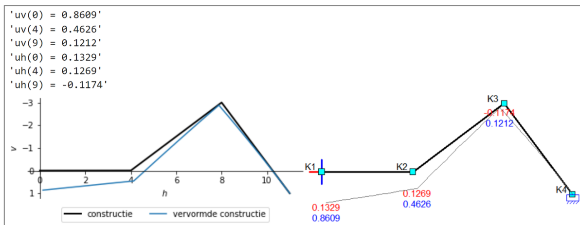
figuur 46: Vervorming van de constructie volgens het model links en volgens matrixframe rechts.
