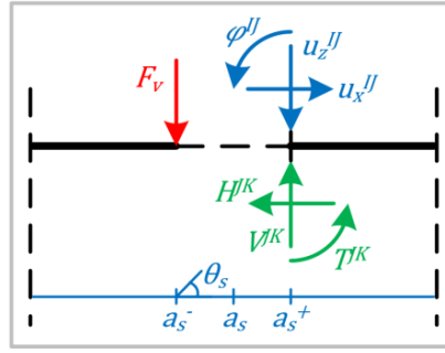
figuur 35: modelleren van een sprongpunt.
