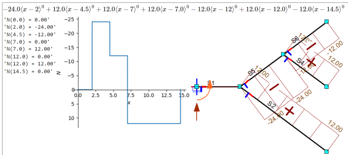
figuur 64: Normaalkrachtenlijn volgens het model links en Matrixframe rechts.
