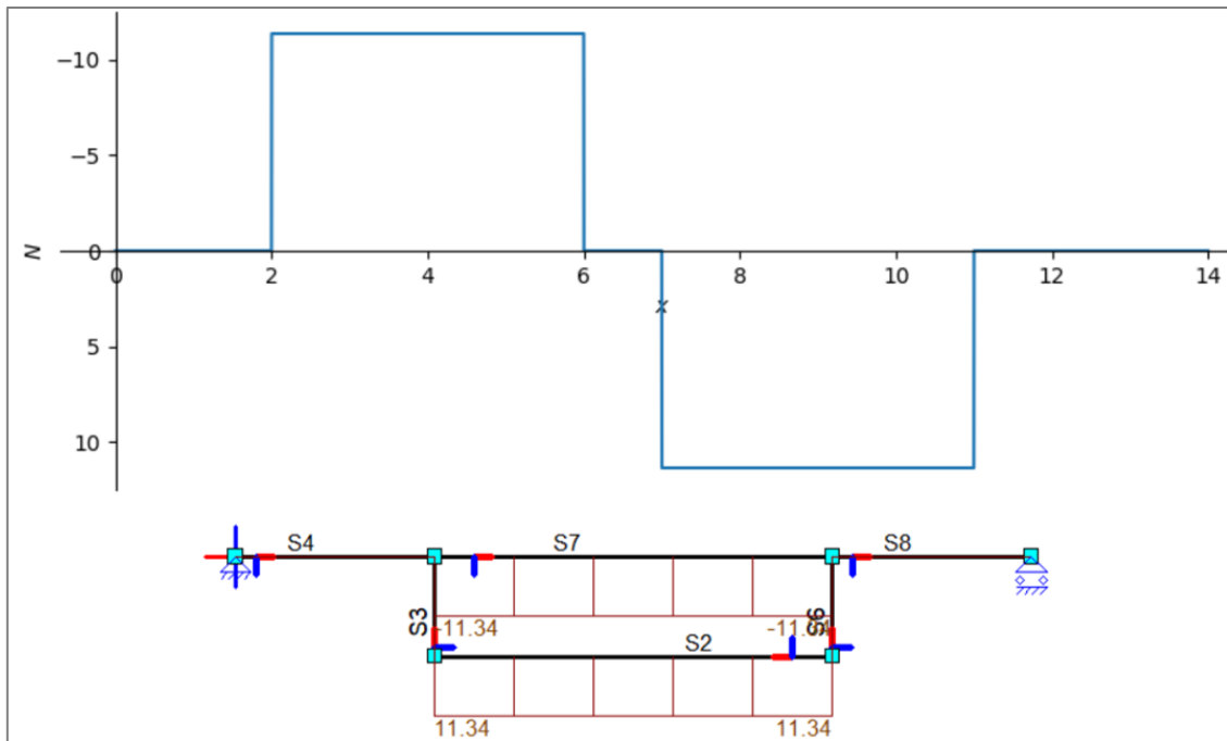
figuur 80: Normaalkrachtenlijn volgens het model boven en Matrixframe onder.
