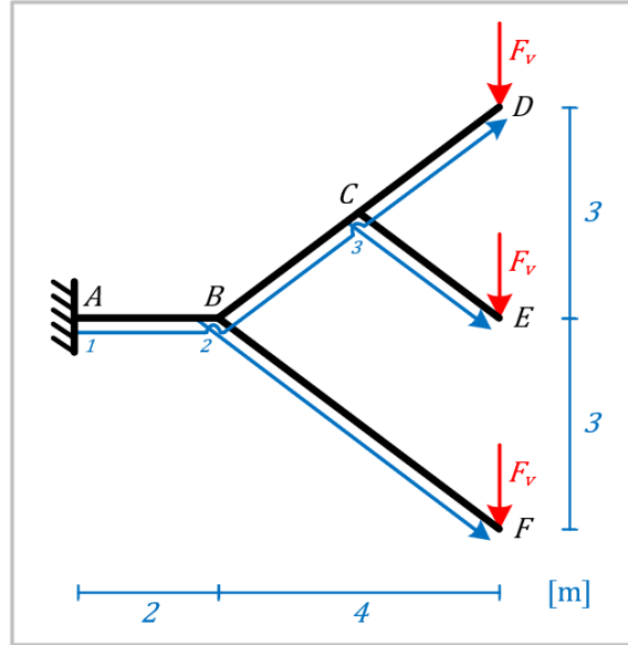
figuur 61: Meermaals vertakte ingeklemde constructie.
