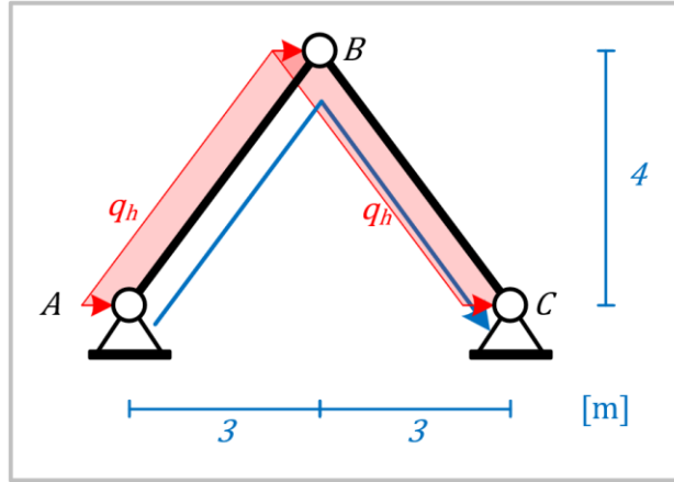
figuur 47: Driescharnierspant.
