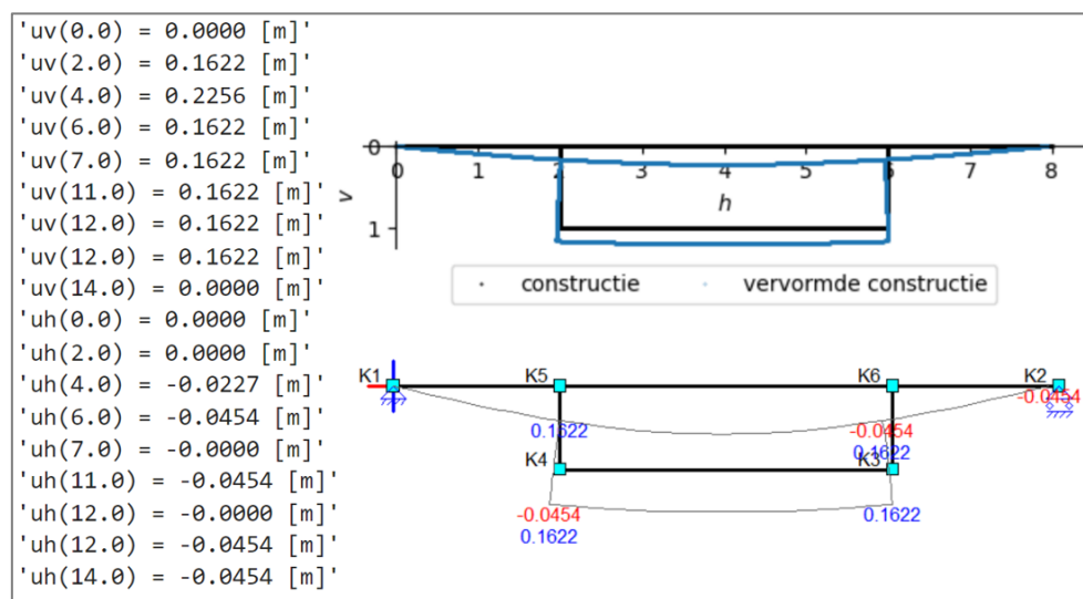
figuur 83: vervormingen volgens het model boven (met de waardes links) en Matrixframe onder.
