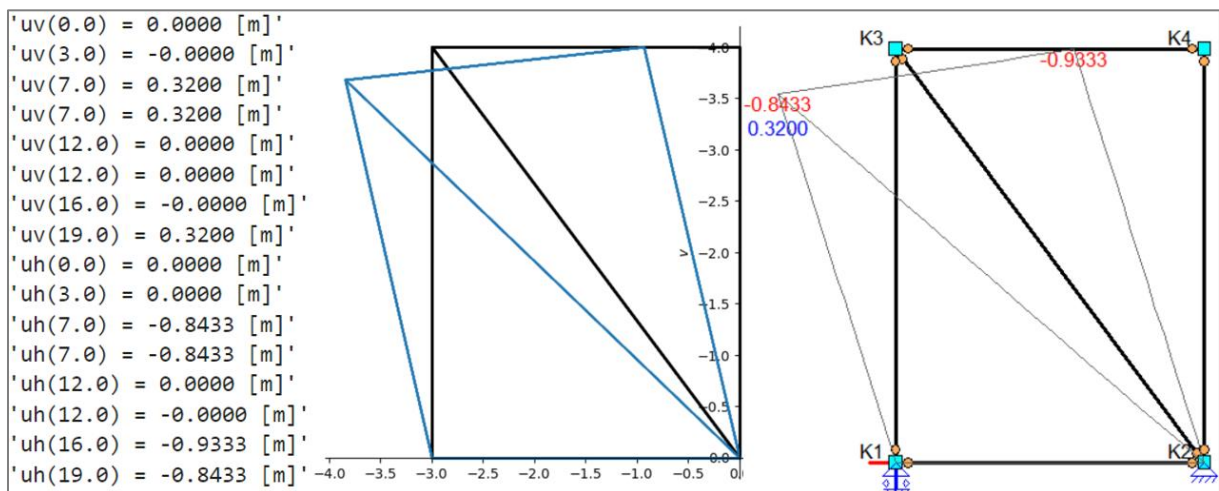
figuur 89: vervormingen volgens het model links en Matrixframe rechts.
