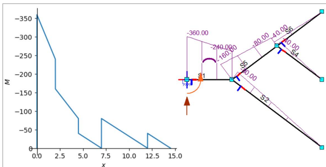
figuur 66: Momentenlijn volgens het model links en Matrixframe rechts.
