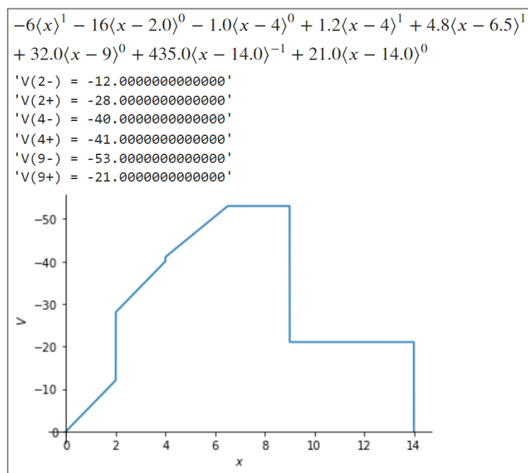
figuur 42: Dwarskrachtenlijn.
