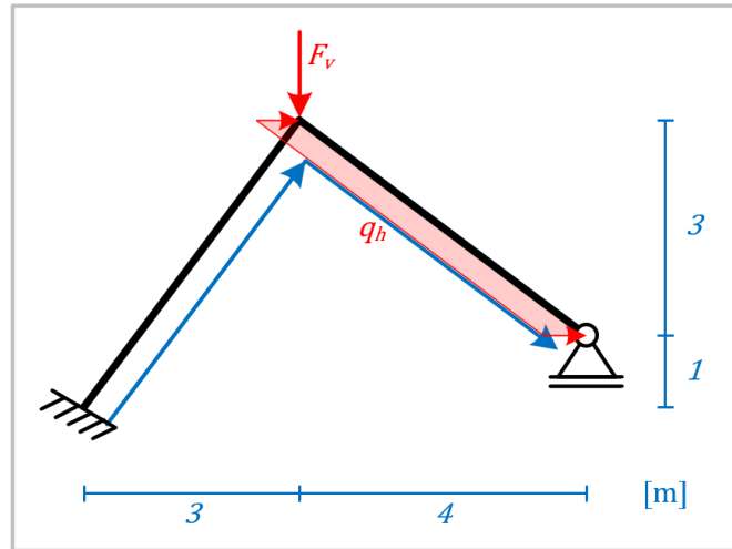
figuur 54: Geknikte Statisch Onbepaalde constructie.
