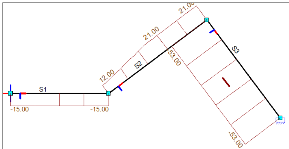
figuur 41: Normaalkrachtenlijn volgens Matrixframe.
