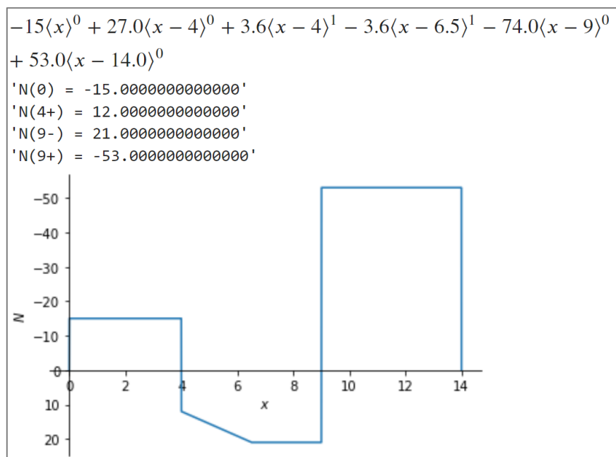
figuur 40: Normaalkrachtenlijn.
