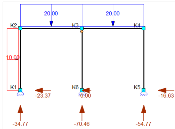
figuur 71: Reactiekrachten in Matrixframe.
