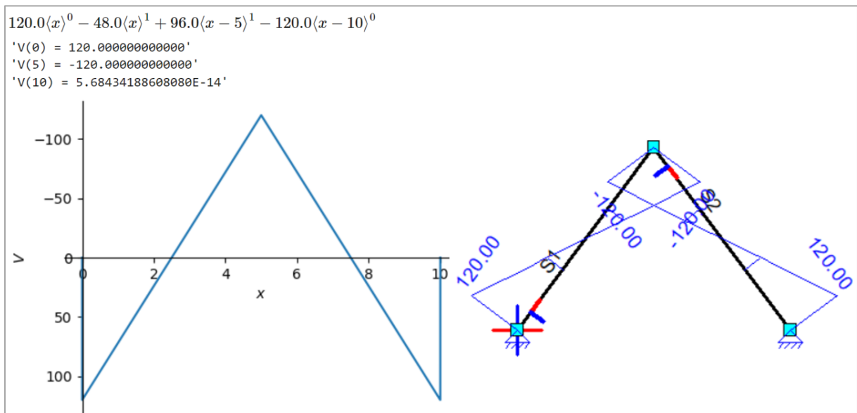
figuur 51: Dwarskrachtenlijn volgens het model links en Matrixframe rechts.
