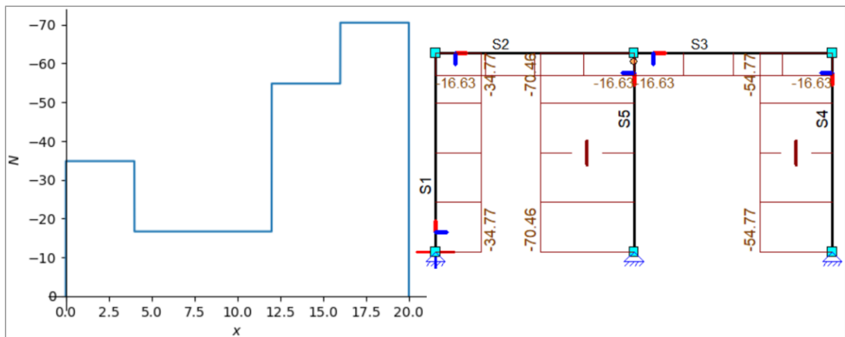
figuur 72: Normaalkrachtenlijn volgens het model links en Matrixframe rechts.
