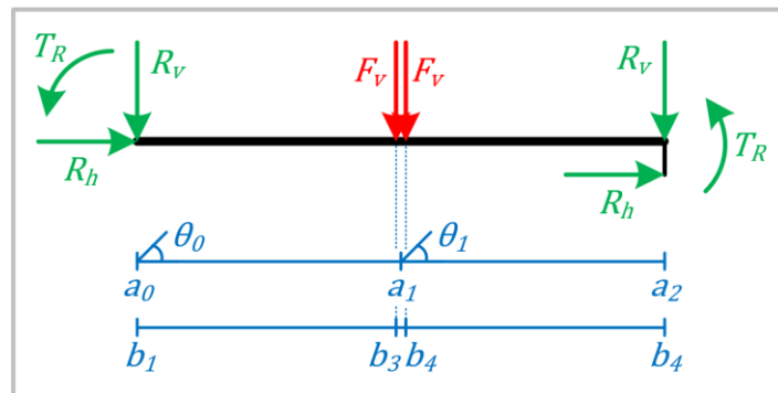
figuur 95: : Gelineariseerde weergave van de constructie in figuur 94.
