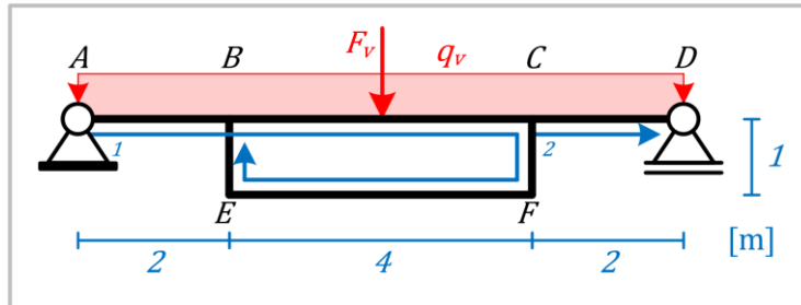
figuur 77: Opgelegde versterkte ligger
