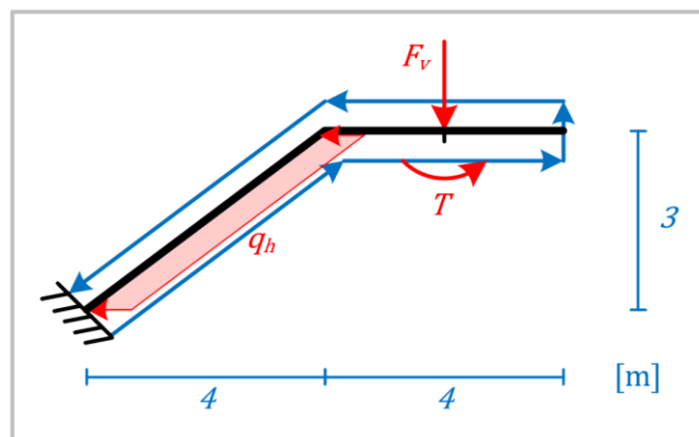
figuur 92: retour over een geknikte constructie.
