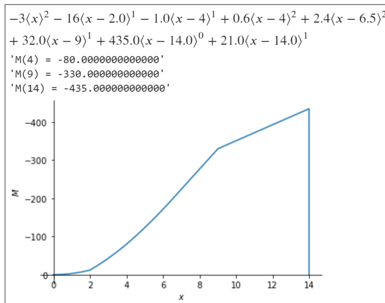
figuur 44: Momentenlijn.
