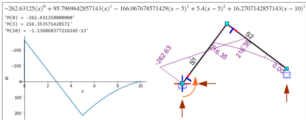
figuur 59: De momentenlijn volgens de Macaulay methode links en Matrixframe rechts.
