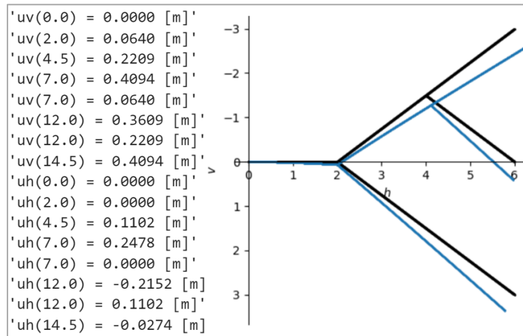
figuur 67: Vervorming volgens het model.
