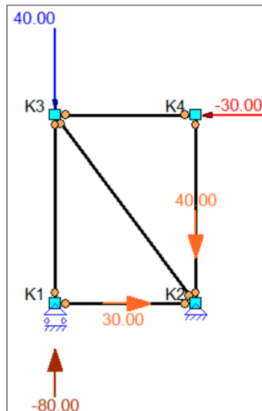
figuur 86: Reactiekrachten in Matrixframe
