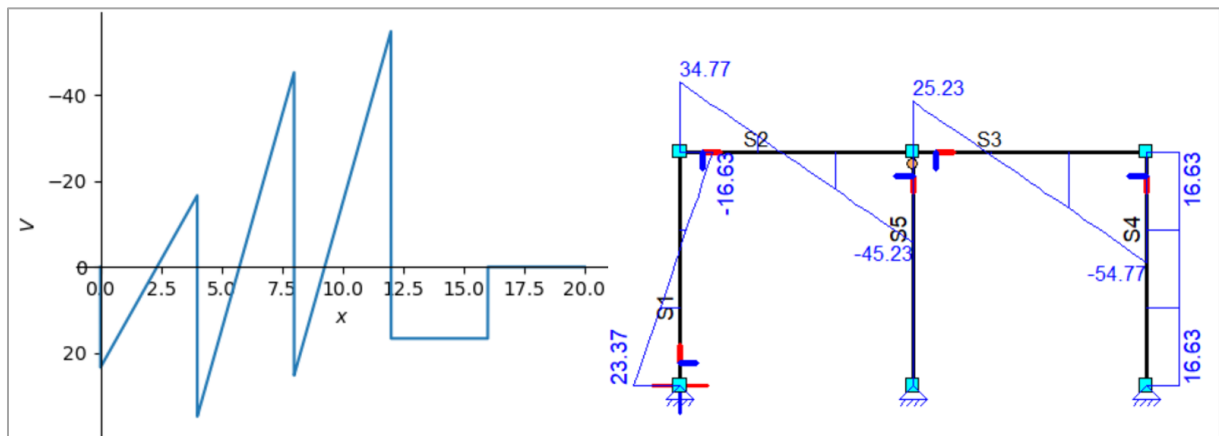
figuur 73: Dwarskrachtenlijn volgens het model links en Matrixframe rechts.
