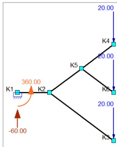
figuur 63: Reactiekrachten in Matrixframe.
