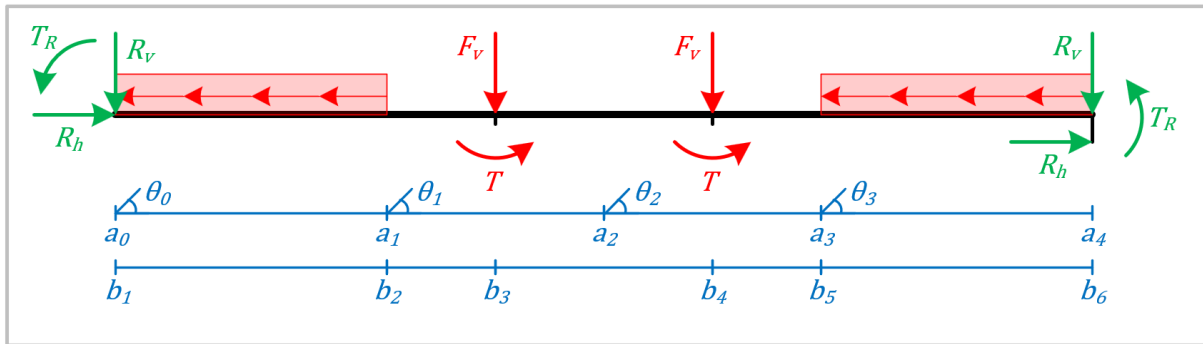
figuur 93: Gelineariseerde weergave van de constructie in figuur 92.
