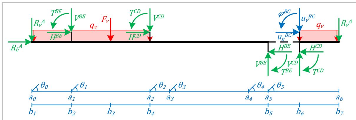
figuur 78: Overzichtsschema behorende bij figuur 77.
