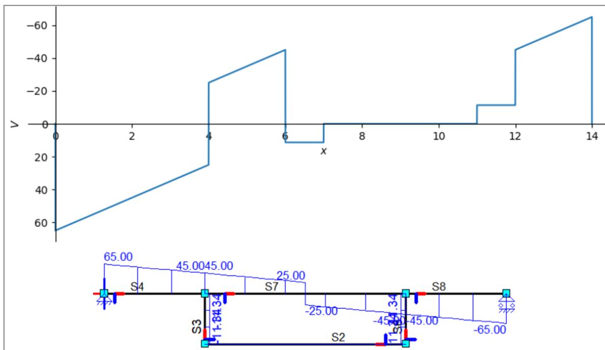
figuur 81: Dwarskrachtenlijn volgens het model boven en Matrixframe onder.
