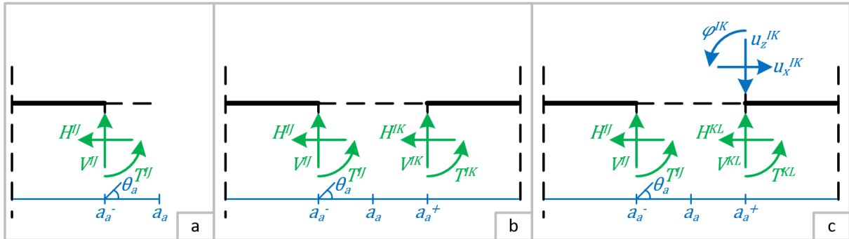
figuur 36: Modelleren van een aansluitpunt als het ook het eindpunt is (a), als de functie erna direct vervolgd (b) of het als het ook een sprongpunt is (c).
