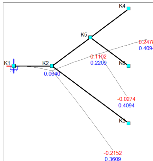
figuur 68: Vervorming volgens Matrixframe.
