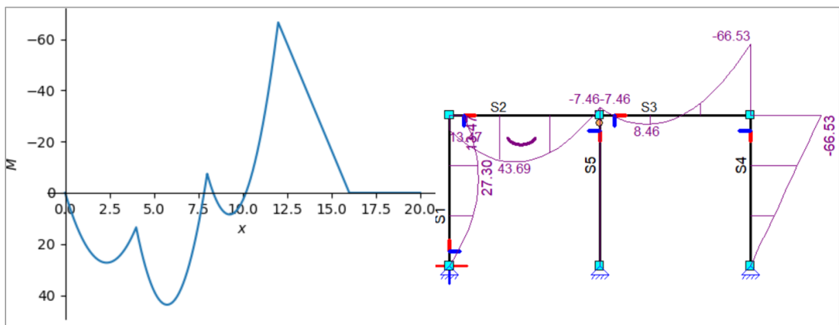
figuur 74: Momentenlijn volgens het model links en Matrixframe rechts.
