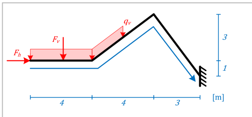
figuur 37: Ingeklemd ligger met twee knikken.
