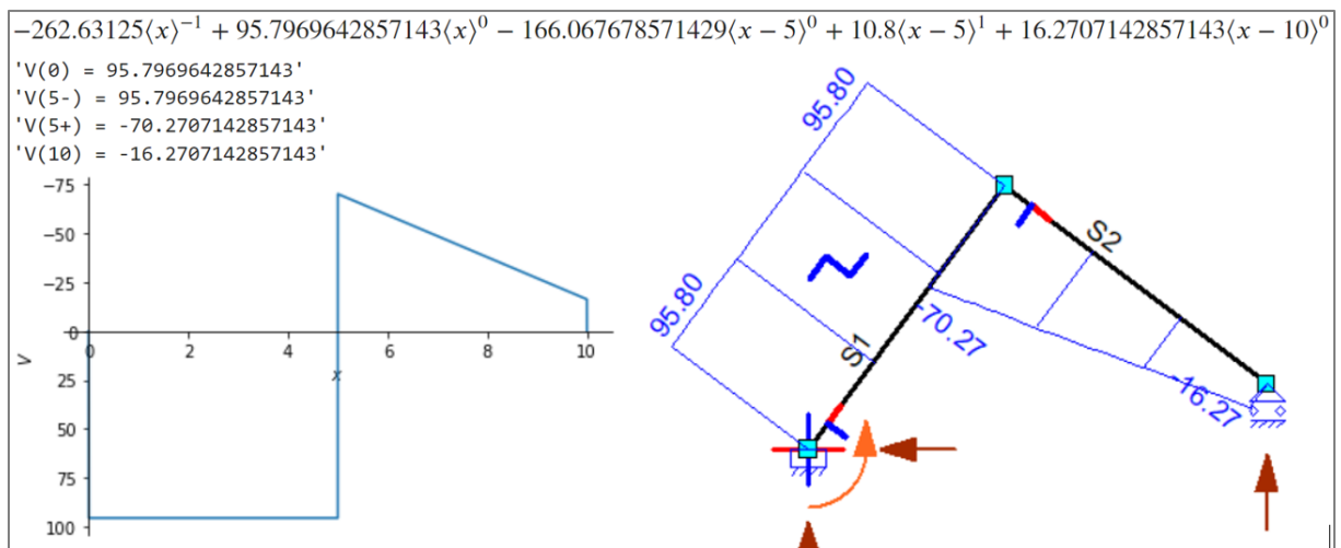
figuur 58: De dwarskrachtenlijn volgens de Macaulay methode links en Matrixframe rechts.
