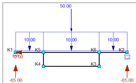
figuur 79: Reactiekrachten in Matrixframe.
