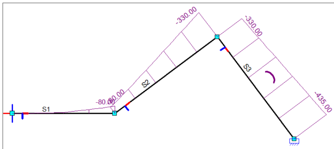
figuur 45: Momentenlijn volgens Matrixframe.
