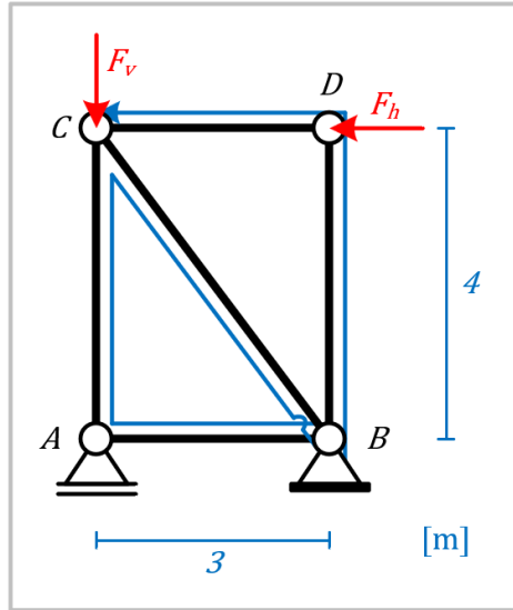
figuur 84: Vakwerk
