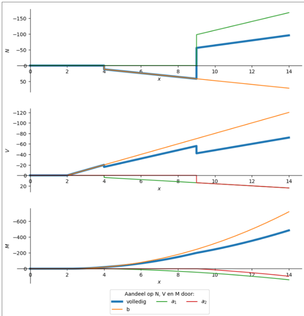
figuur 15: De invloed van de begin- en hoektermen op de volledige snedekracht diagrammen van de uniforme verdeelde belasting in figuur 13 geplot over de lokale as.
