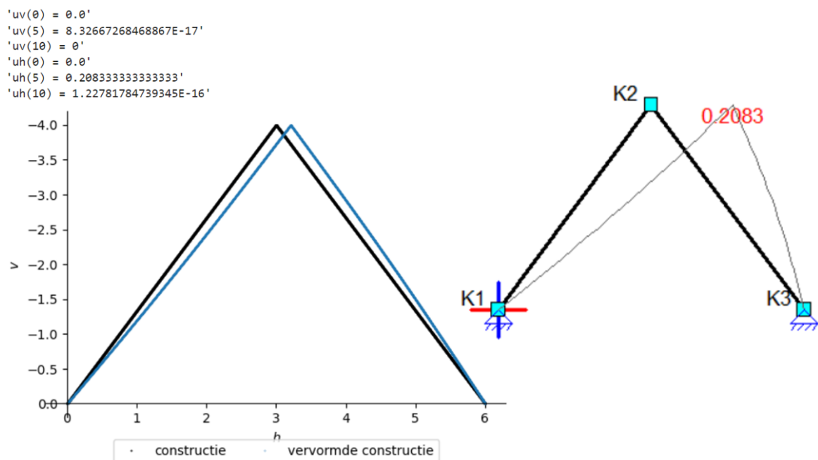
figuur 53: Vervorming van de constructie volgens het model links en volgens matrixframe rechts.
