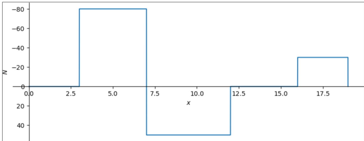
figuur 87: Normaalkrachtenlijn volgens het model.
