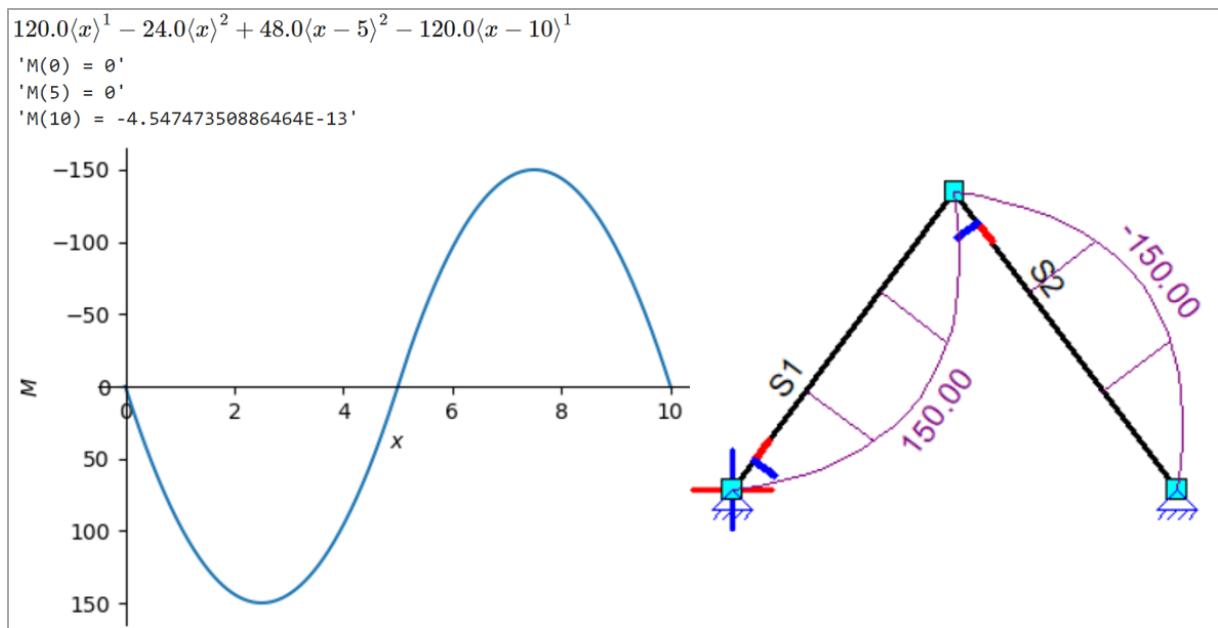
figuur 52: momentenlijn volgens het model links en Matrixframe rechts.
