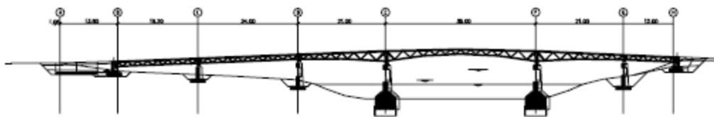
Fig.Ap3.21. Longitudinal section
